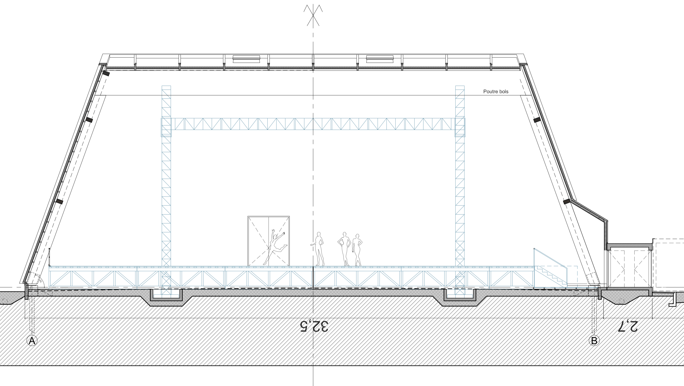
COUPE LONGITUDINALE
